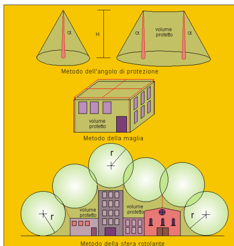
Figura 4 – I tre metodi per la determinazione del volume protetto
