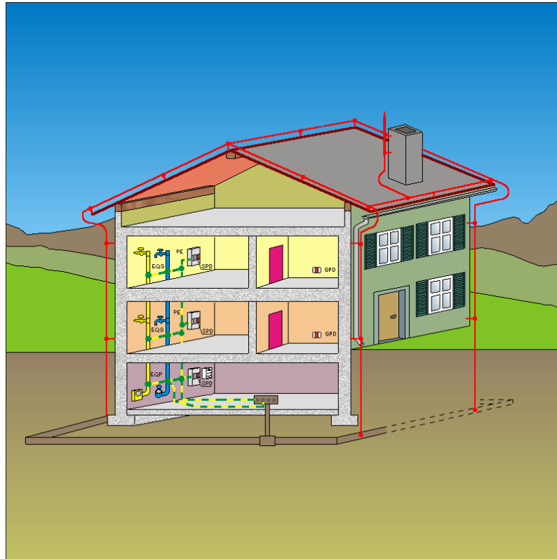
Figura 8 – Principali componenti di un Lps interno
