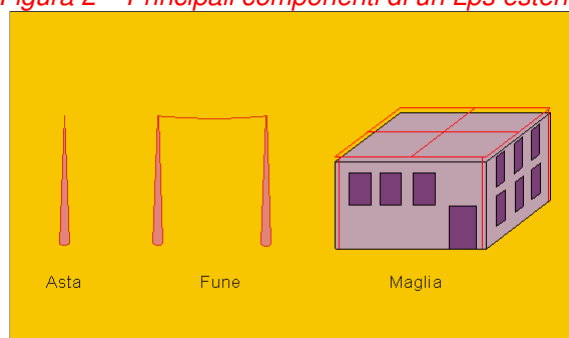
Figura 3 – I tipi di captatori previsti
