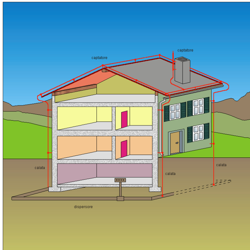
Figura 2 – Principali componenti di un Lps esterno
