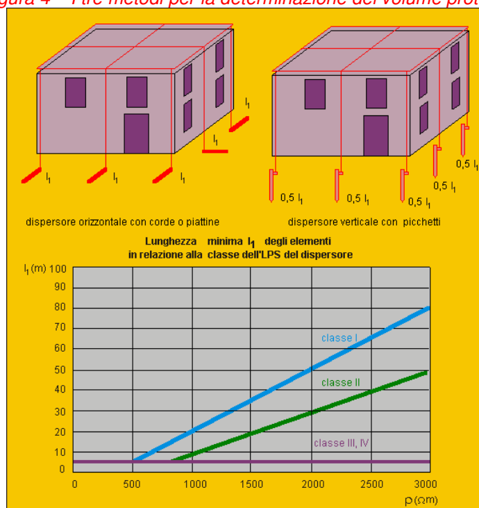
Figura 6 – Dispersore di tipo A
