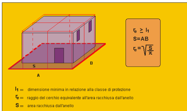
Figura 7 – Dispersore di tipo B
